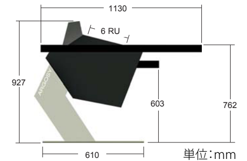
Mirage AWS 900+ Dimensions
