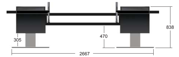
Mirage AWS 900+ Dimensions
