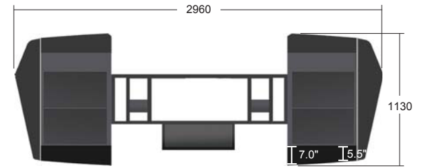
Mirage AWS 900+ Dimensions
