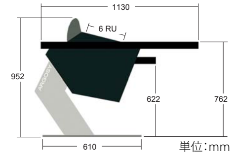
Mirage DC and NCJ24 Dimensions
