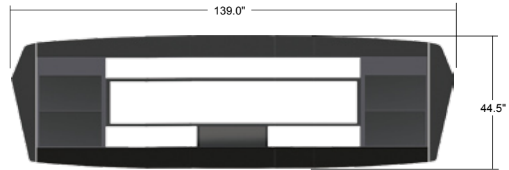
Mirage DC40 Dimensions
