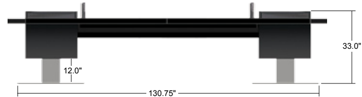
Mirage DC40 Dimensions
