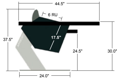
Mirage DC Dimensions
